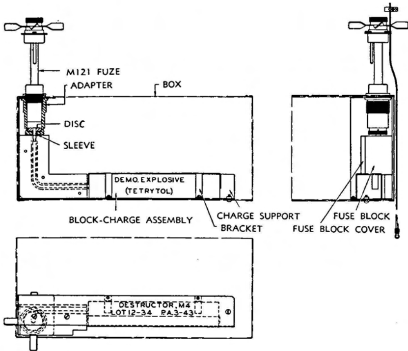
Fig. 218. M4 destructor.
