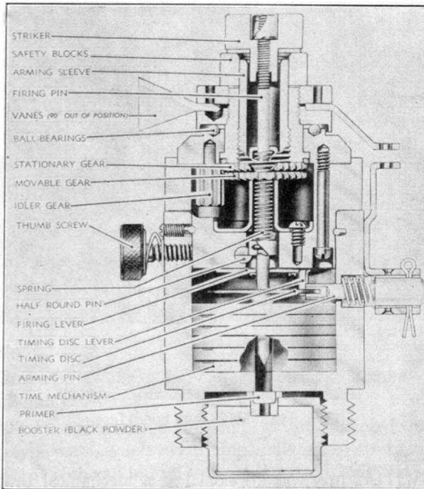
FIG. 143. M111A2 nose bomb fuze.
