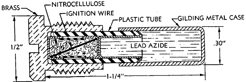
FIG. 215. M1 destructor.
