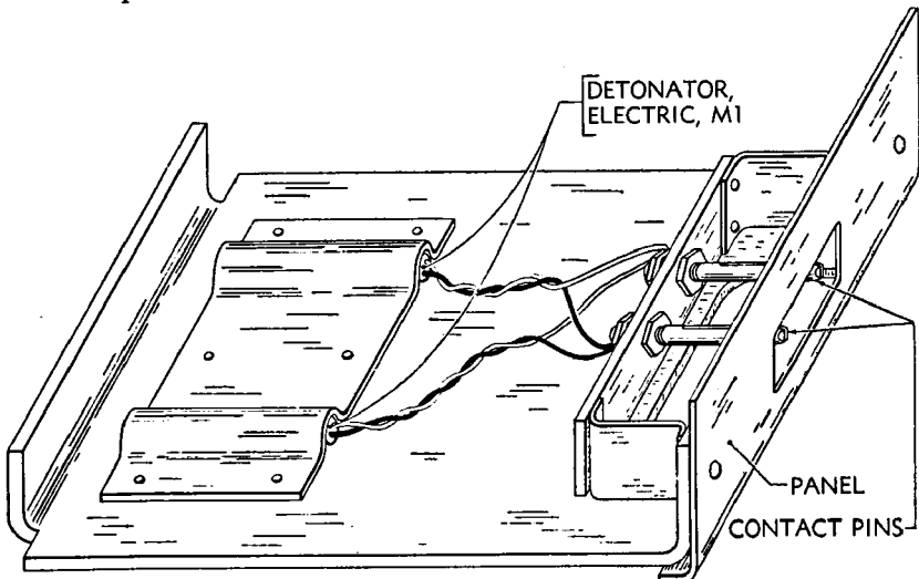
FIG. 216. M2 destructor.
