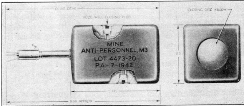
FIG. 213. Demolition-type antipersonnel mine.
