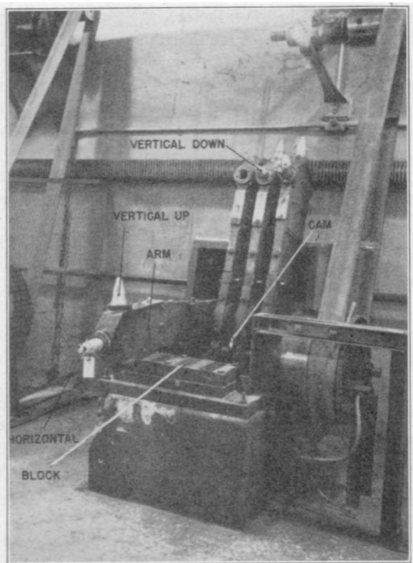
FIG. 54. Jolt machine.
