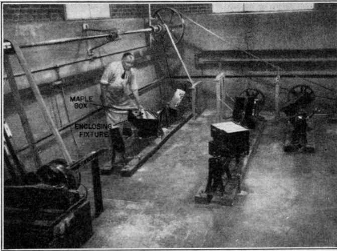
FIG. 55. Jumble machine.
