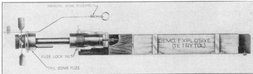
FIG. 219. M5 destructor.
