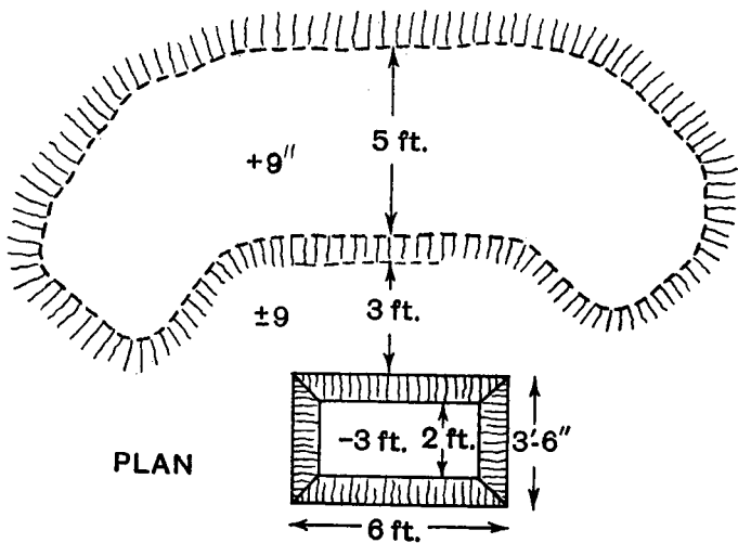
FIG. 18.—Emplacement.
