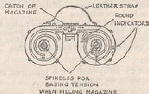
GERMAN M.G. 15.
