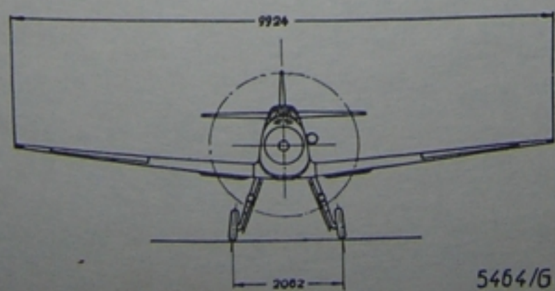
Abb. 2: Flugzeugmusterblatt
